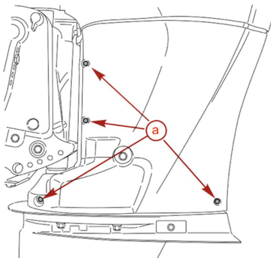
a - Vis arrière du carénage du carter moteur (4)
