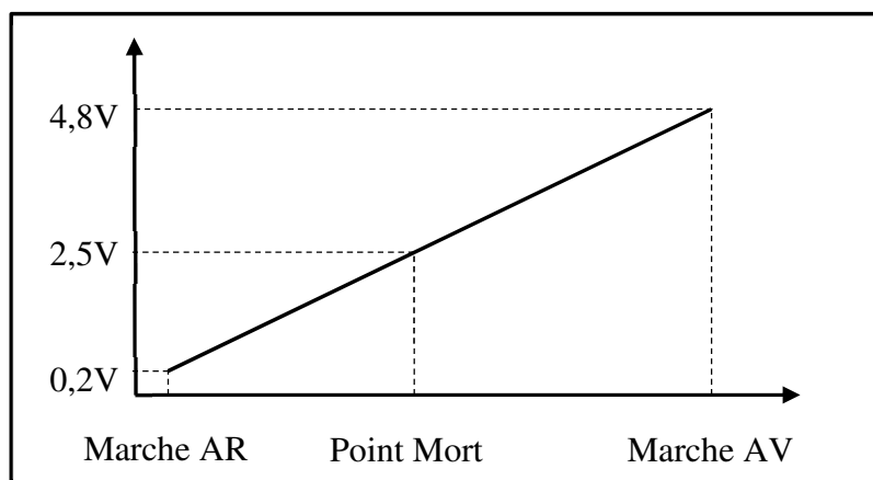
Schéma de tension du signal de position de marche
