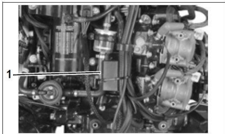
1. Module de relais de soupapes d'échappement
