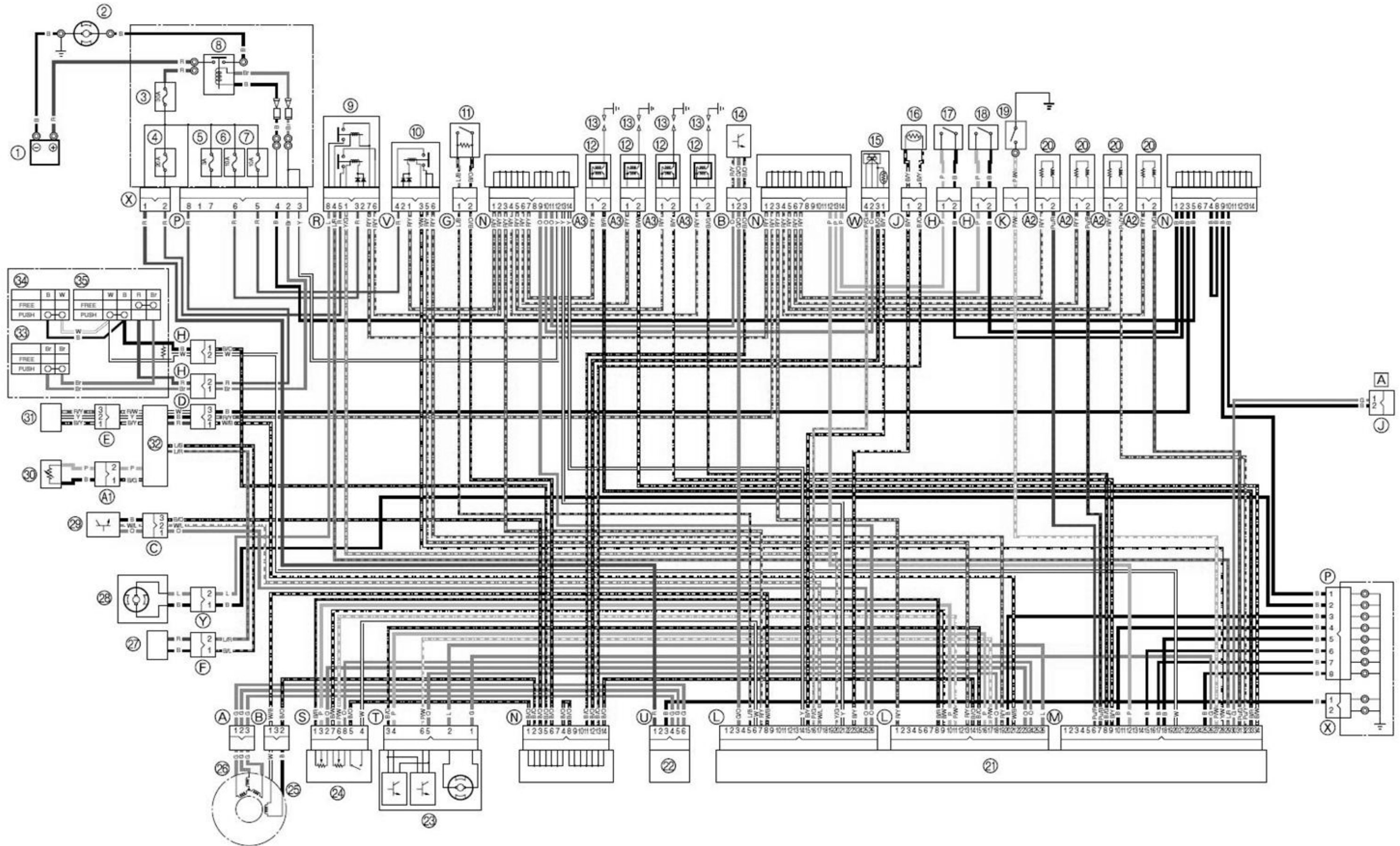
DR 8. Schéma électrique du Yamaha VX 110 Sport
